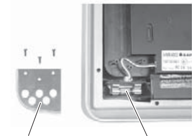
Metallabdeckung
