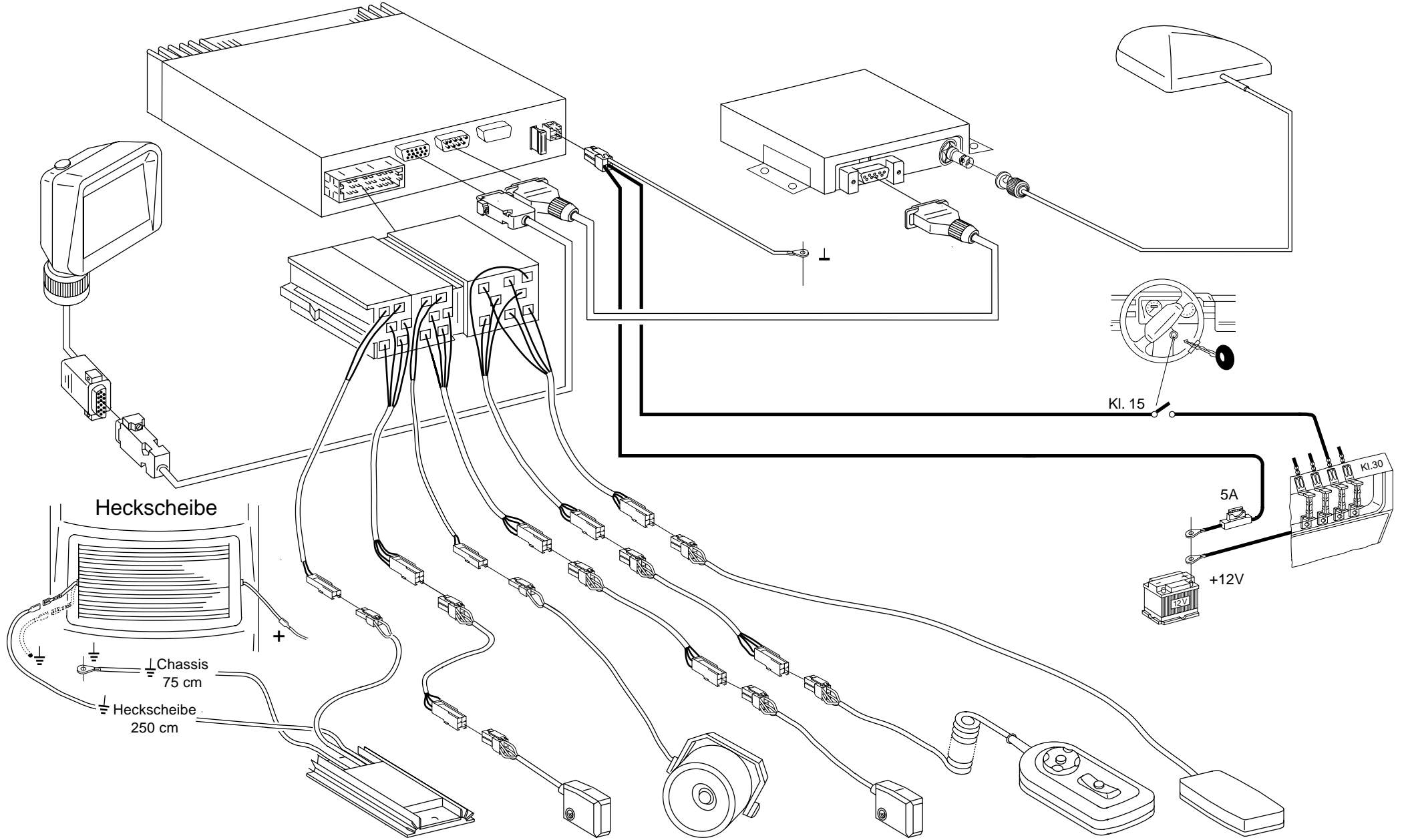
Anschluß der Sensoren Fig. 11
